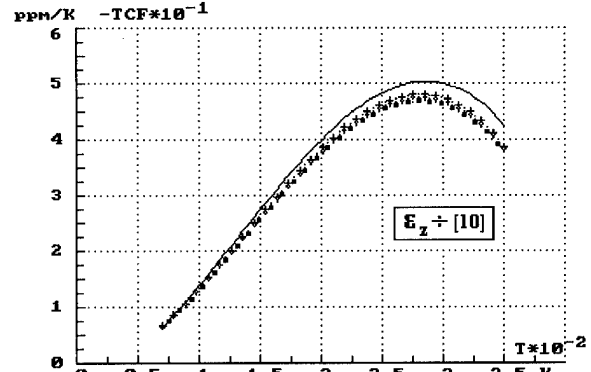
Fig. 6. Sapphire DDR TCF(T):
